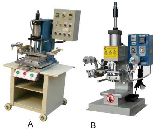
ZU-142 气压式烫金机 Pneumatic Hot Stamping Machine
